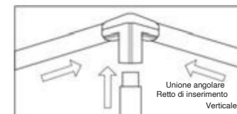
Metodo di installazione per i 4 angoli
