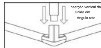
Método de instalação dos quatro tubos de espuma de canto.
