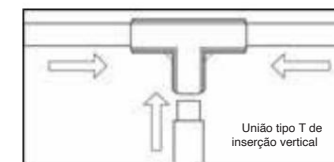
Método de instalação intermediário
