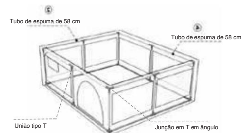
Resultado final da instalação concluída.
