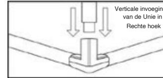
Installatiemethode van de vier hoekschuimbuisen.
