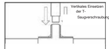
Vertikales Einsetzen der T-Saugverschraubung
