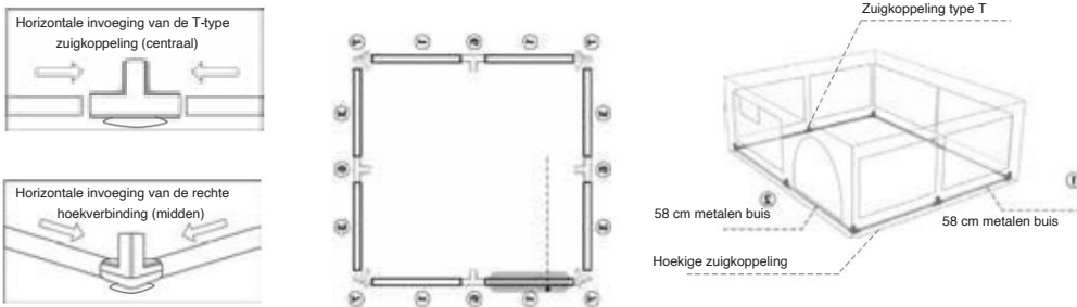
Gevolg van het voltooiën van de installatie van het onderste frame
