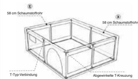
Endergebnis der abgeschlossenen Installation.
