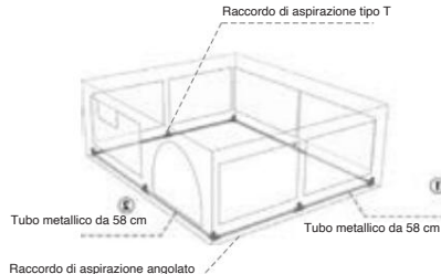
Effetto del completamento dell'installazione del telaio inferiore
