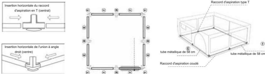
Effet de l'achèvement de l'installation du cadre inférieur
