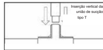
Método de instalação de tubos de espuma intermediários.
