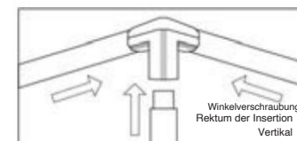
Installationsmethode für die 4 Ecken
