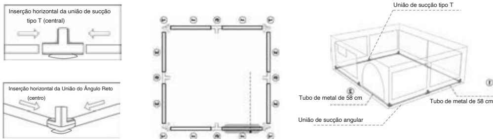
Efeito da conclusão da instalação da estrutura inferior
