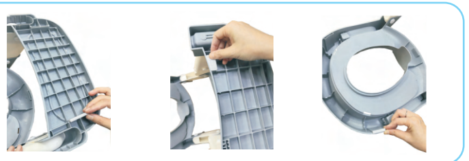
6. Alle rutschfesten Gummis in die vorgesehenen Schlitz einbauen.
